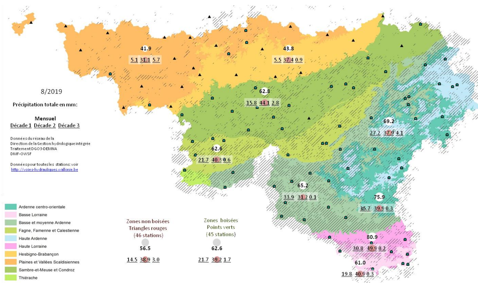
Comparaison des précipitations totales (mm) par décade et par mois, en moyenne par région bioclimatique dans les zones boisées et comparaison chiffrée pour les zones boisées et non boisées de toute la région, sur base des données du réseau de la direction de la gestion hydraulique intégrée-DGO2 et du réseau CRAW-PAMESEB.
